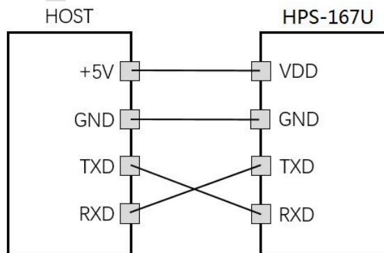
图3 HPS-167U的连接方式
