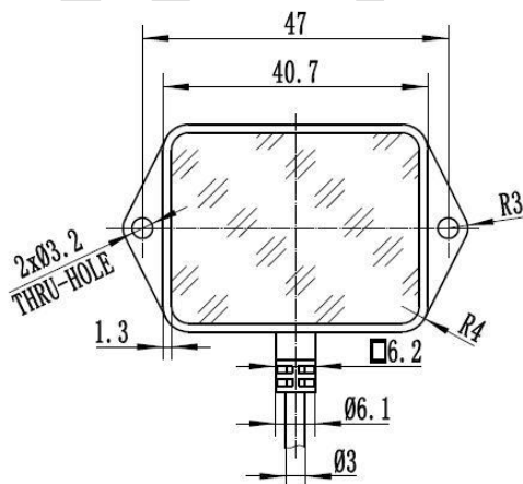
图 1. HPS-167U 前视图
