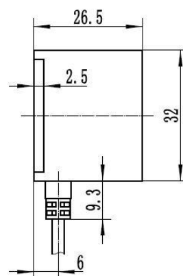
图 2. HPS-167U 侧视图
